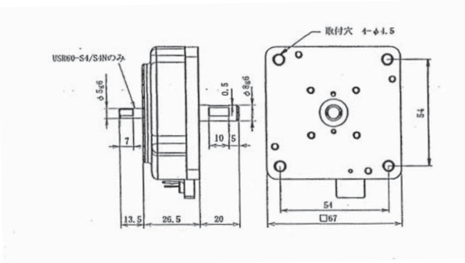
USR60-S3/S4/S3N/S4N の外形図
