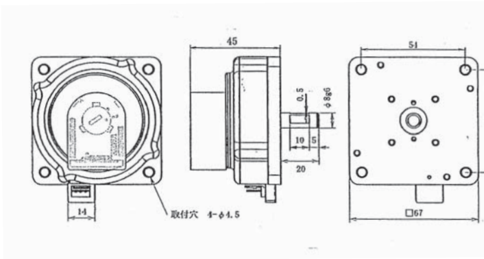
USR60-E3/E3T/E3N/E3NT の外形図
